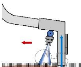
Système par injection extraction
